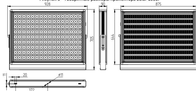
Рисунок 4 – Габаритные размеры прожектора Solar 1500 с поворотным кронштейном.
